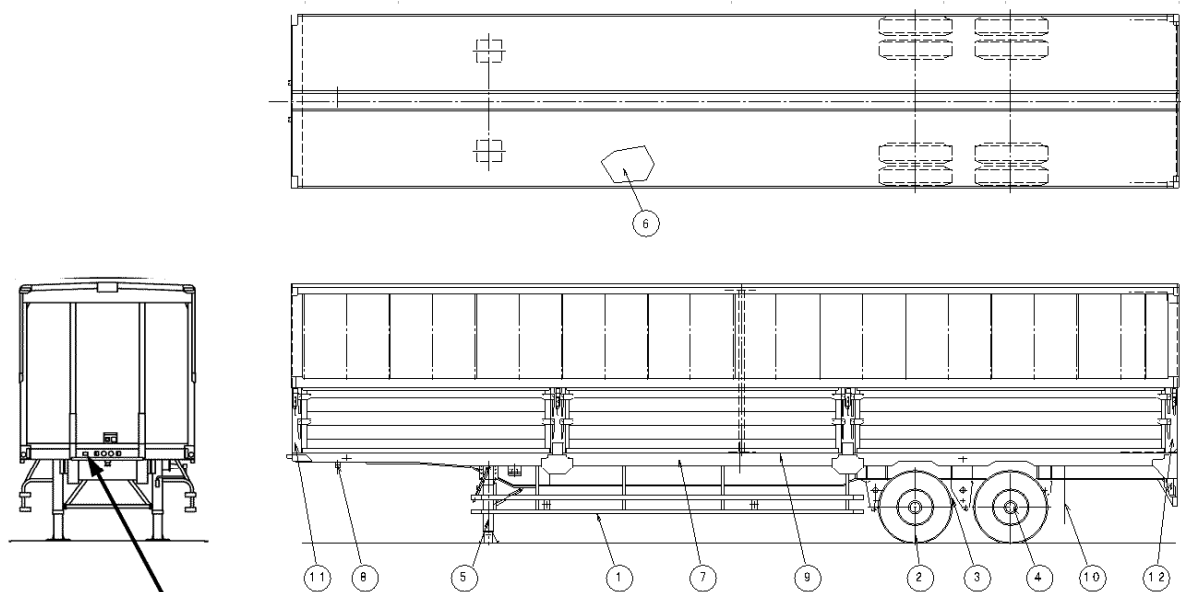
製造銘板例
