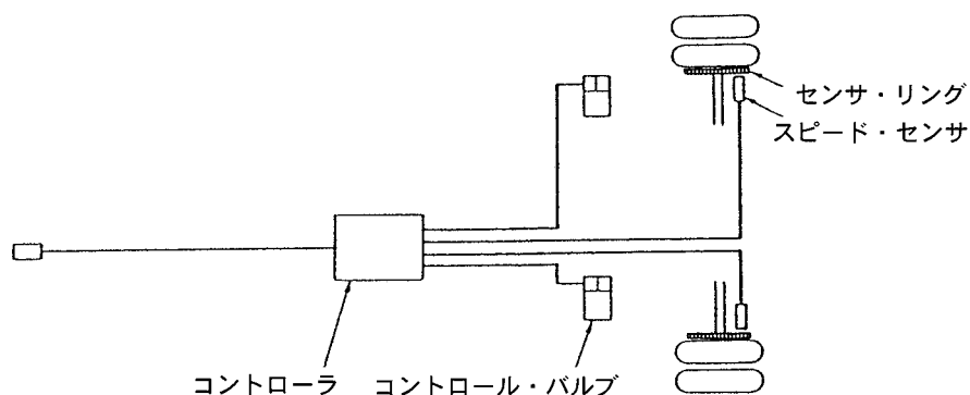
ABS 用電気配線図
