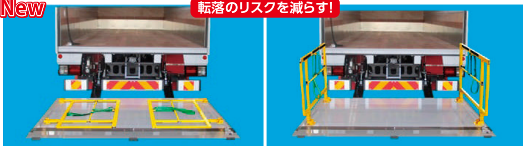
▶ 安全柵 注1
