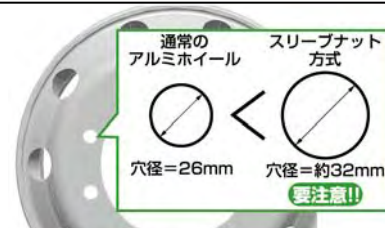
スリーブ・ナット方式用アルミ・ホイール
