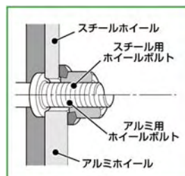
シングルタイヤの例
