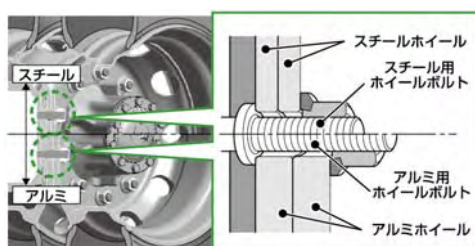
ダブルタイヤの例
