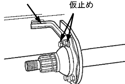
シェイドプレート
