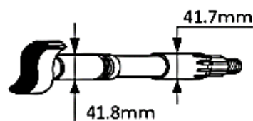
カムシャフト新品寸法
