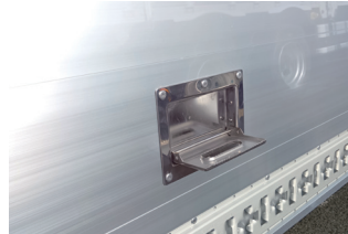
アオリステップ格納式
