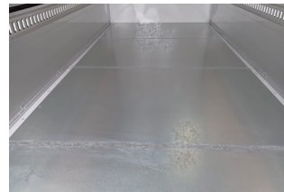
床ライニング (全面) 亜鉛鉄板 t=2.3
