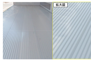
フロアリング アルミ形材 t=22 ローレット
