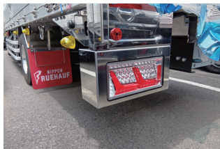
テールランプ BOX 吊下 SUS #400
