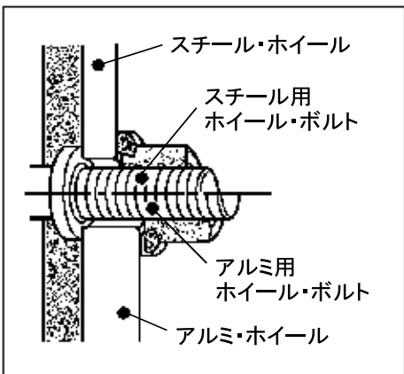
シングル・タイヤの例
