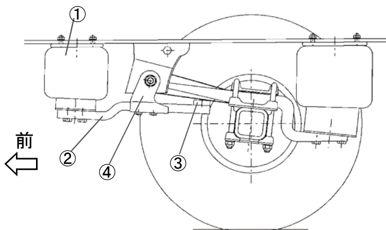
後前軸を下げた状態
