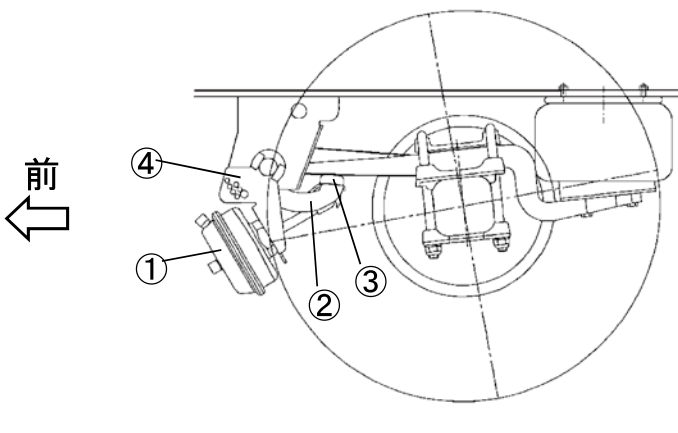
後前軸及び後々軸を上げた状態
