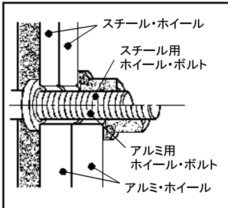
ダブル・タイヤの例
