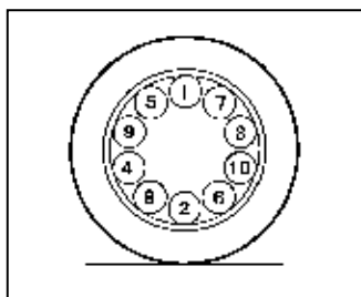
ホイール・ナットの締付け順序
