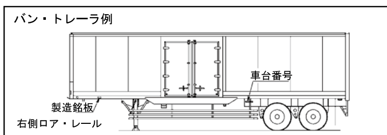
製造銘板の例
