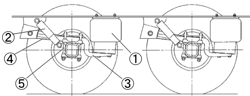
2 軸 車
