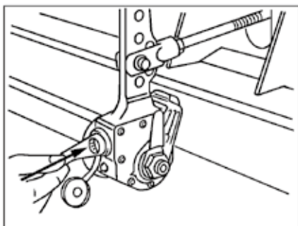
調整ねじを回す
