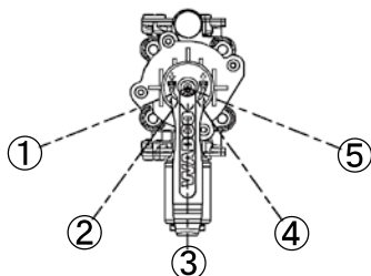
ハイット・コントロール・レバー 位置図
