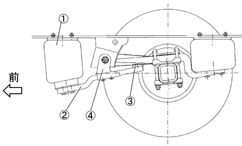
後前軸を上げた状態
