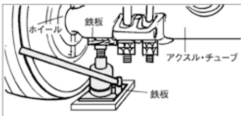
ジャッキ・アップ
