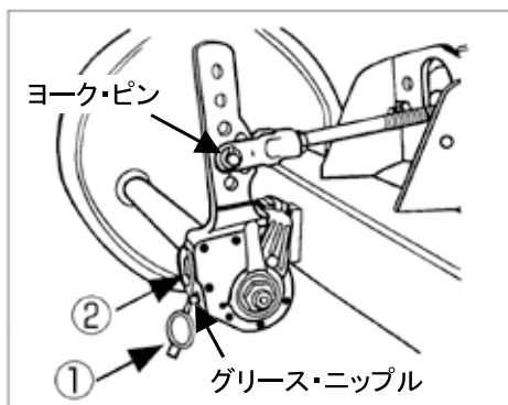
SMBアクスル用
