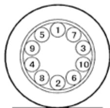
ISO方式締め付け順 (10本ボルト式)
