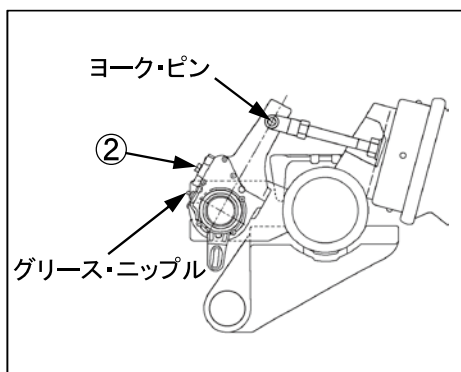
FUWAアクスル用
