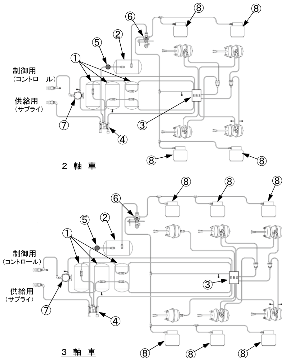
主要部品表
