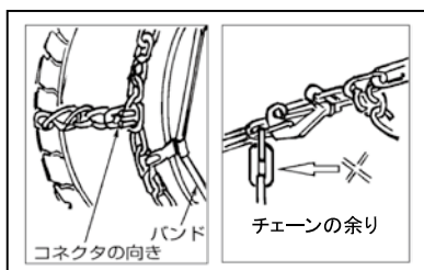
タイヤチェーンの装着
