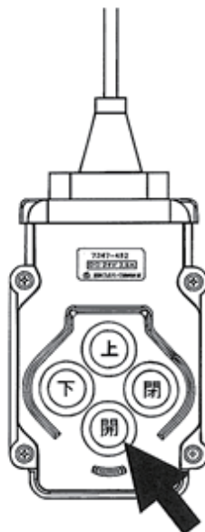
スイッチボックス内ペンダント スイッチでの操作
