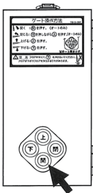
スイッチボックスでの 操作
