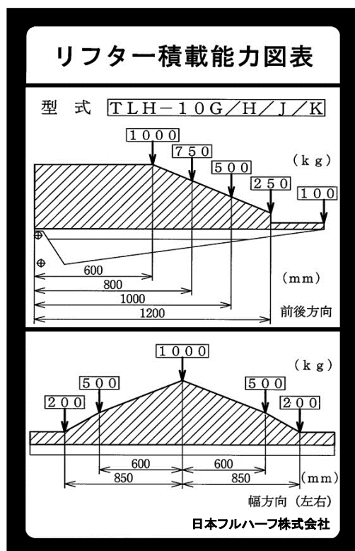
リフター積載能力図表
